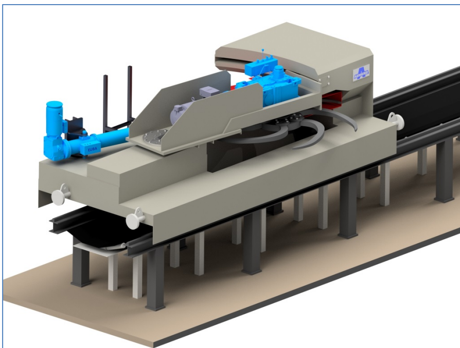
AUMUND-Bunkerentleerungswagen BEW-FLS Typ LOUISE (Illustration ©AUMUND)
