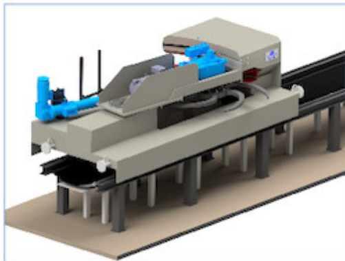
AUMUND Bunkerentleerungswagen BEW-FLS Typ LOUISE (Illustration ©AUMUND)
