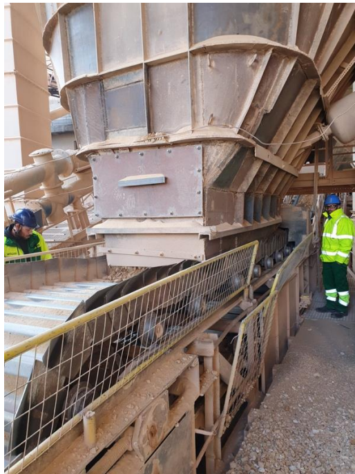
AUMUND-Buckelplattenband in Volos/Griechenland (Referenz-Anlage, Foto AUMUND)
